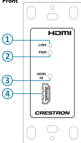
HD-TX-4KZ-101-1G, Front
