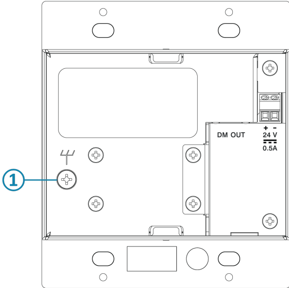
HD-TXU-4KZ-111-2G, Rear
