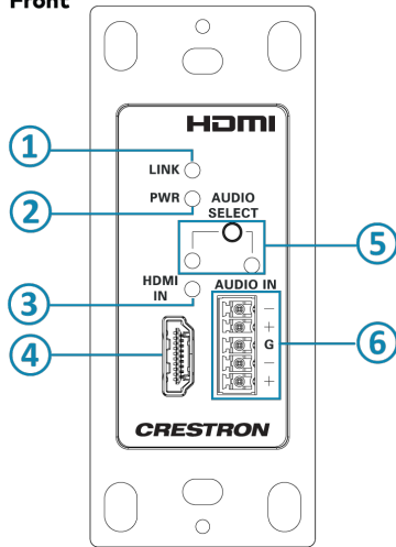
HD-TXA-4KZ-101-1G, Front
