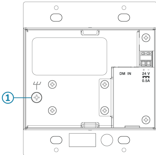
HD-RXU-4KZ-101-2G, Rear
