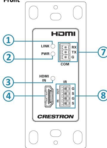
HD-TXC-4KZ-101-1G, Front
